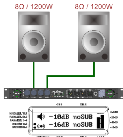
x2 橋接輸出分別接 1 隻 8\Omega 喇叭 預估最大輸出：1200Wx2
