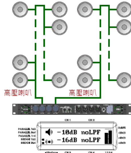
x2 橋接輸出分別接 1 堆並接的高壓喇叭 預估最大輸出：600Wx2
