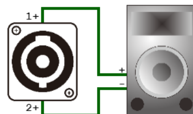
橋接（BTL）
