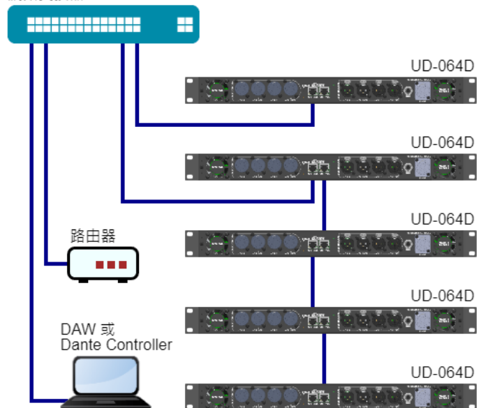
網路交換器
