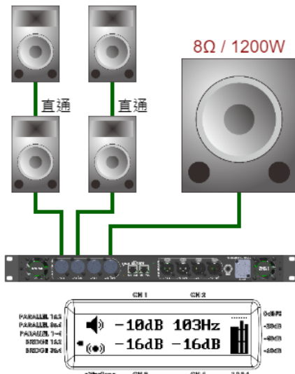
x3 輸出 (混搭 x1 組橋接及 x2 單端) 預估最大輸出：1200W + 600Wx2
