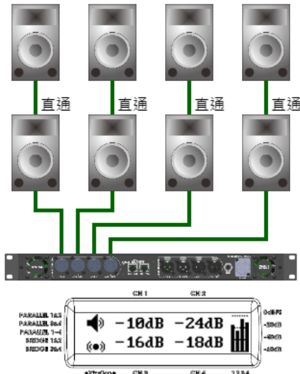
x4 單端輸出分別接 1 組並接喇叭 預估最大輸出：600Wx4
