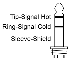
TRS 平衡式插頭接法
