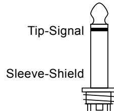
TS 非平衡式插頭接法
